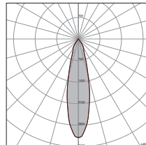
Ottica ST 25°
