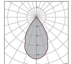
Ottica LA 50°
