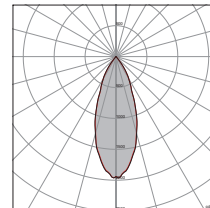
Ottica MD 38°
