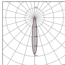
Ottica SP 16°
